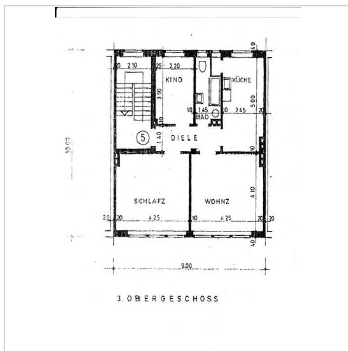
Grundriß
